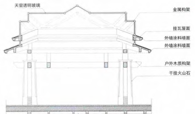
入口门厅剖面大样
