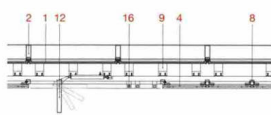
西立面陶板双层幕墙墙身详图
