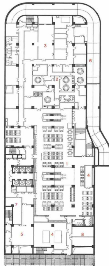
地下一层平面 0 5 10 20m
