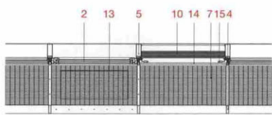
南立面绿植墙墙身详图 0 0.5 1 2m
