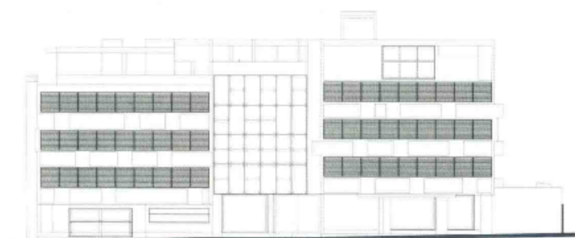
东立面图
