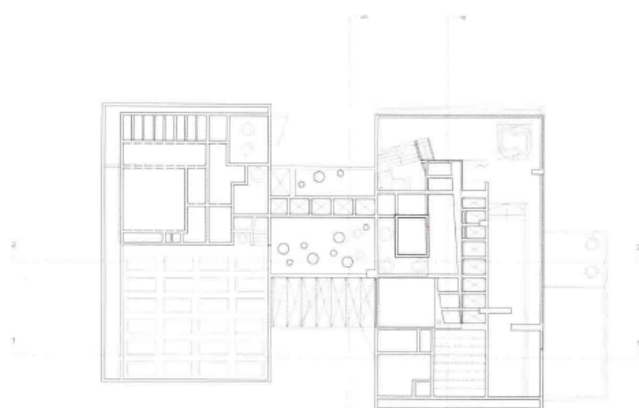
五层平面图
