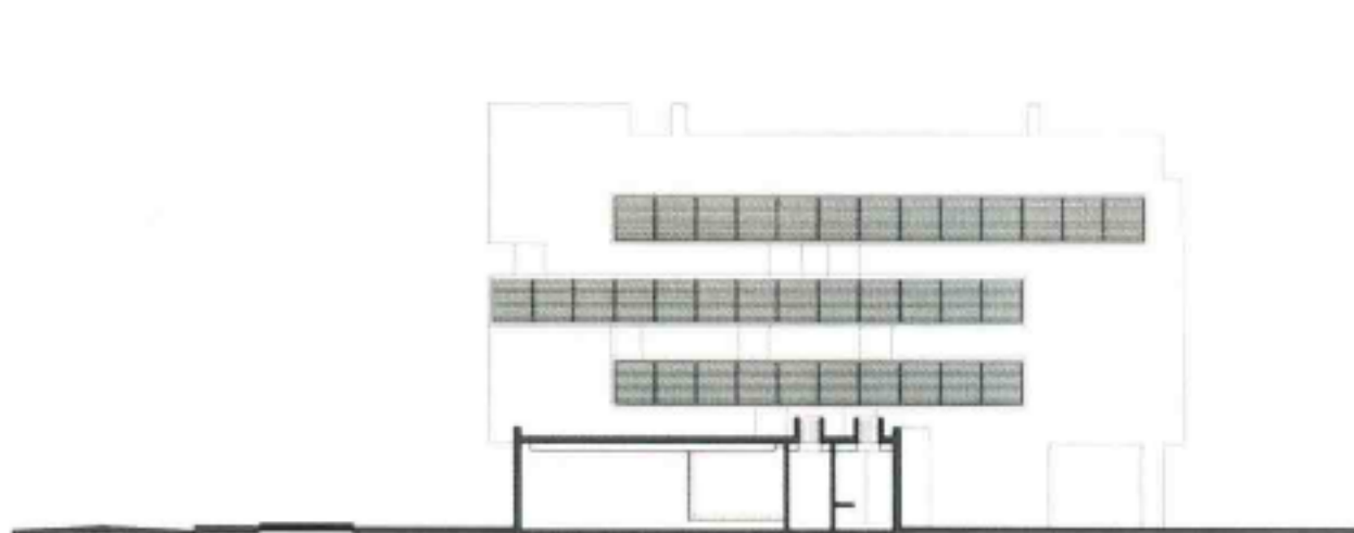
北立面图
