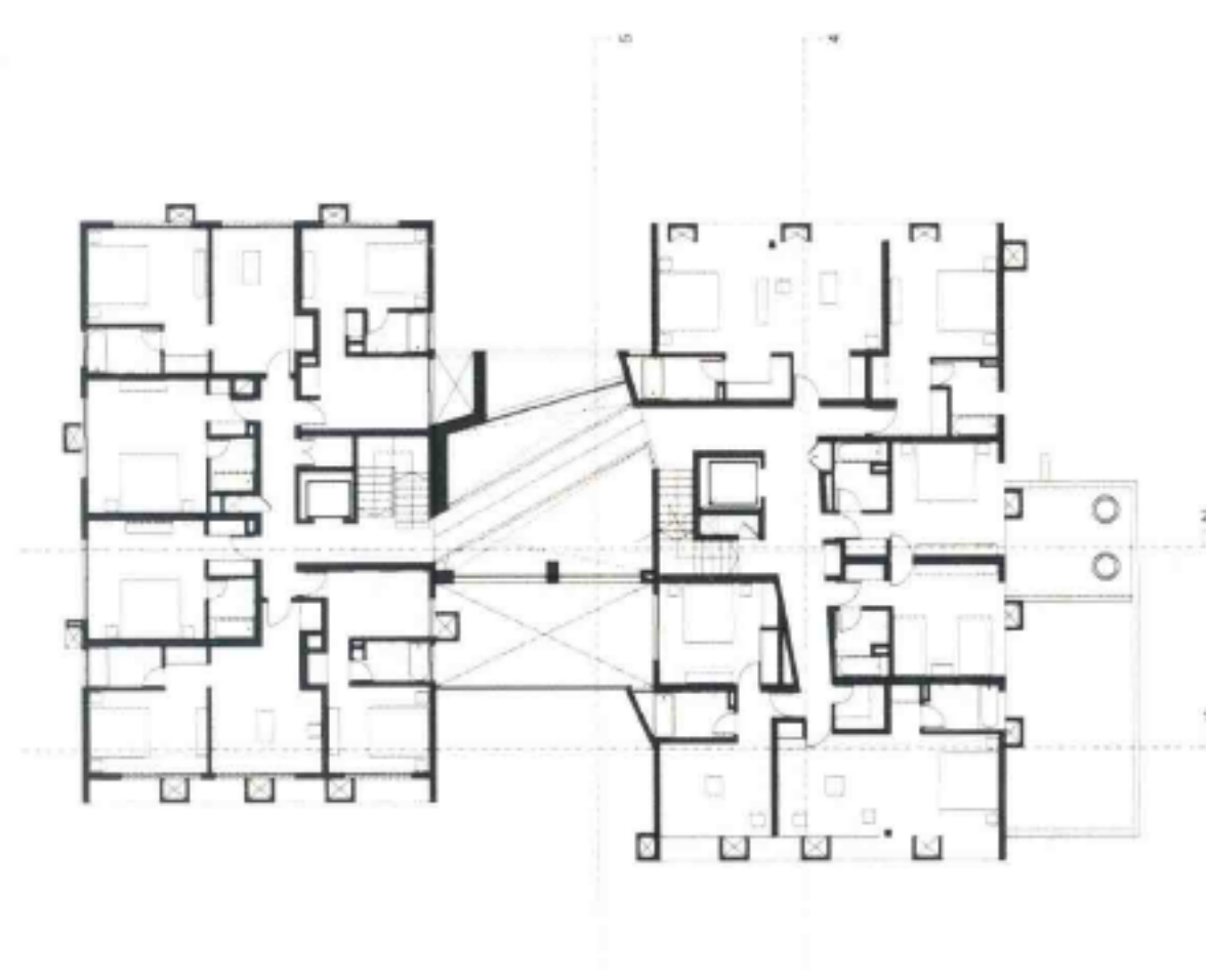
三层平面图
