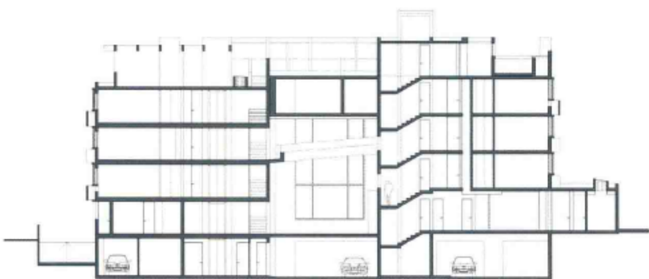
剖面图1-1
