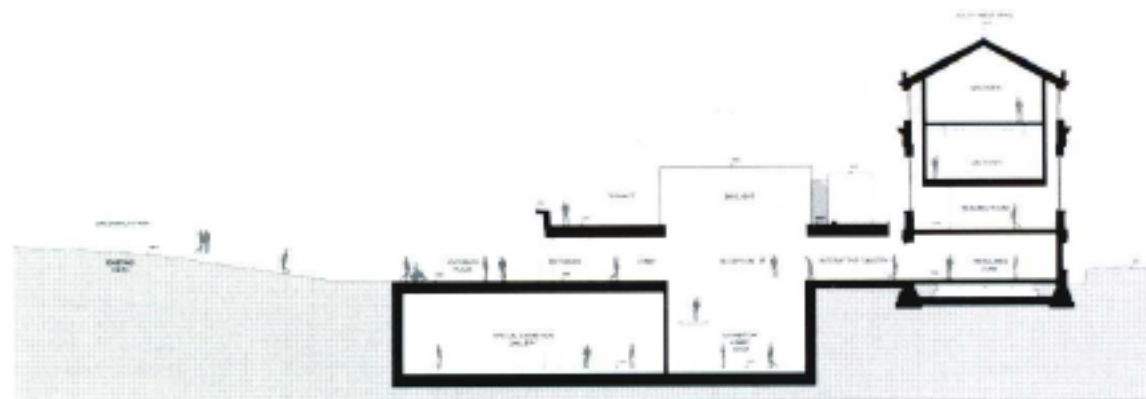
剖面图 B-B
