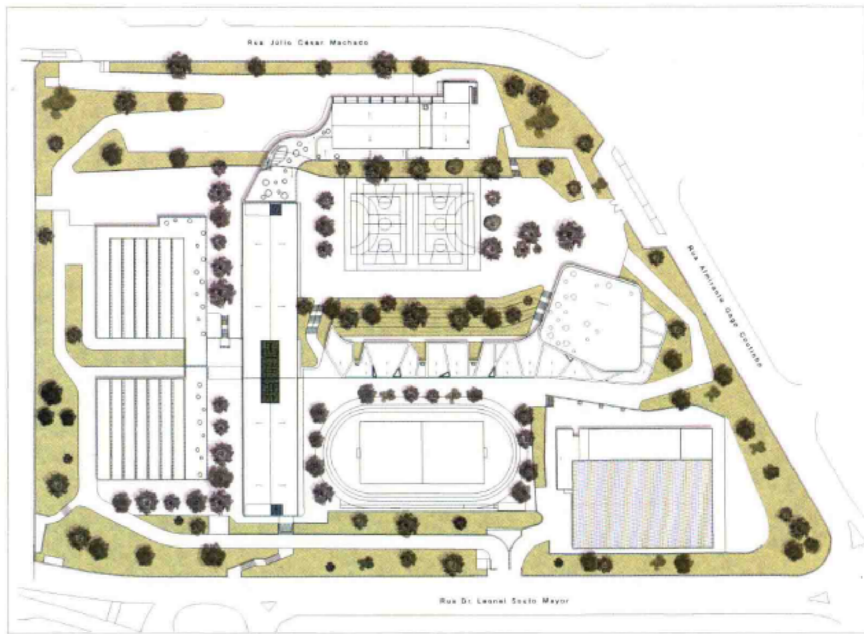
总平面图
