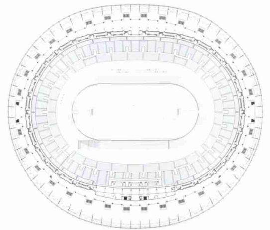
19.7m 标高观众入口层平面 0 10 20 50m
