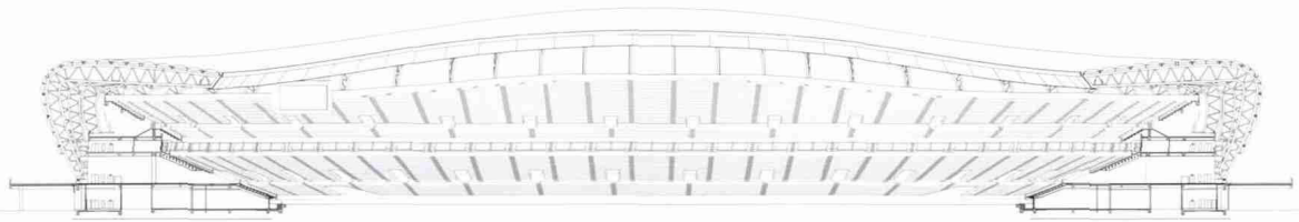
剖面 0 10 20 50m
