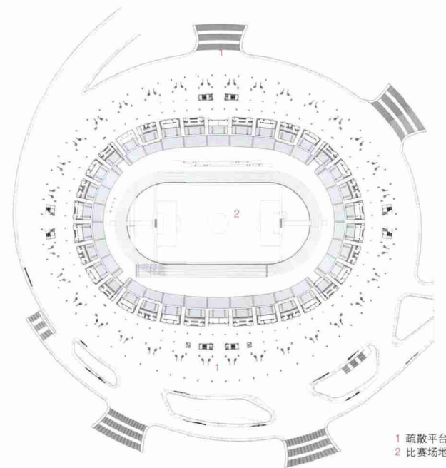
6.95m 标高观众入口层平面 0 10 20 50m
