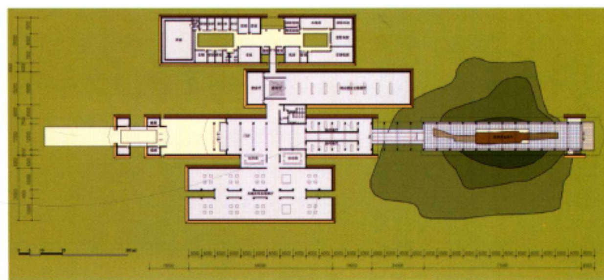
一层平面图
