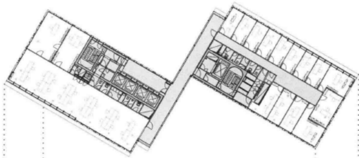
34. OBERGESCHOSS
