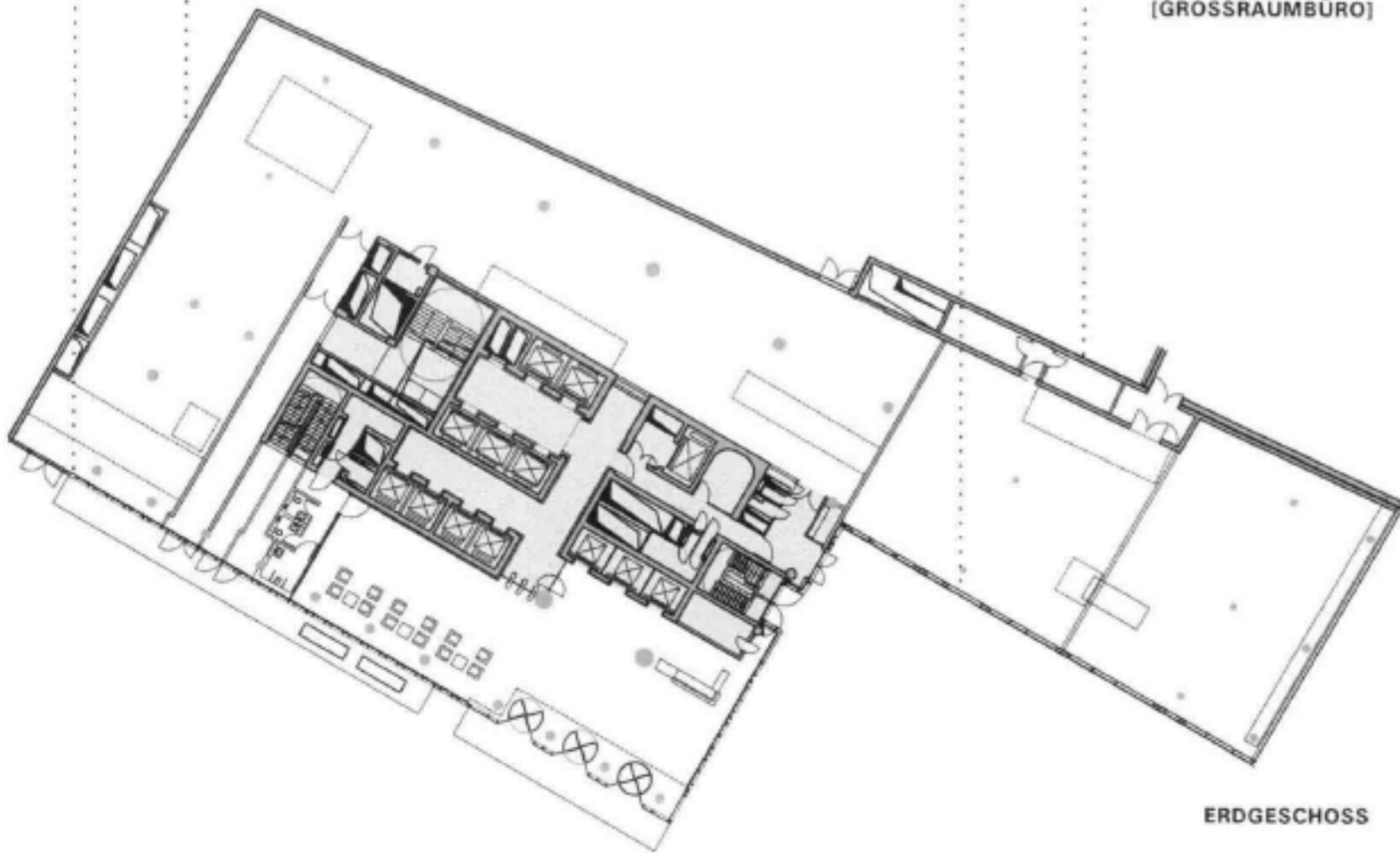
REGELGESCHOSS [GROSSRAUMBÜRO]
