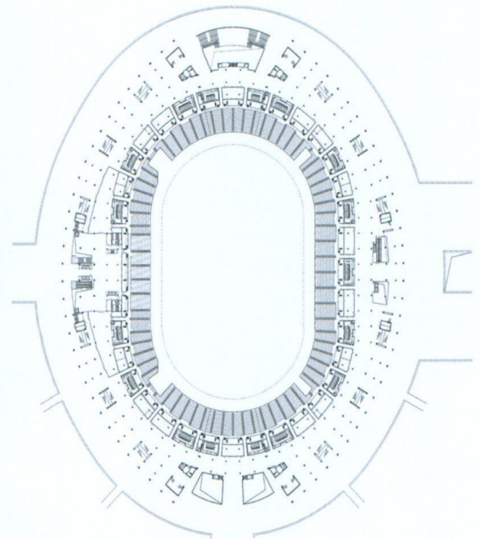
体育场二层平面
