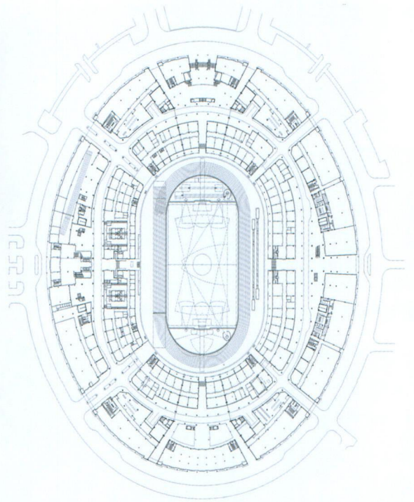
体育场一层平面
