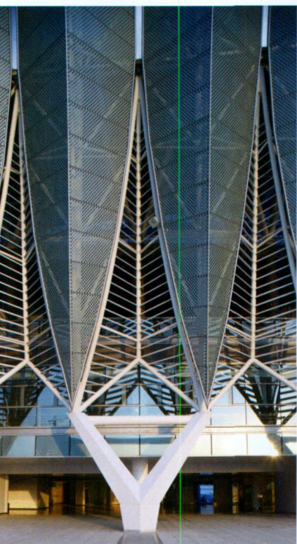
体育场罩棚立面局部
