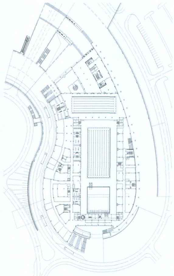
游泳馆平面
