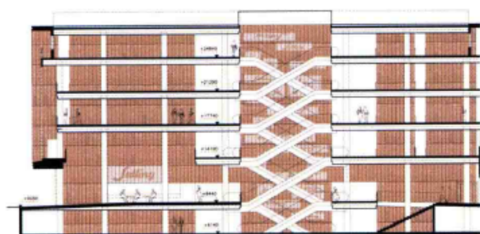
中庭剖面图
