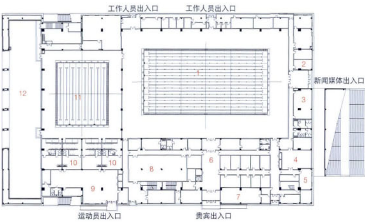
游泳馆一层平面 0 5 10 20m
