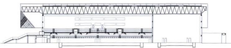
游泳馆剖面 0 5 10 20m
