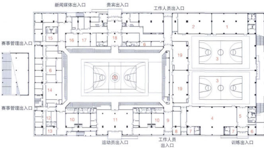
体育馆一层平面 0 5 10 20m
