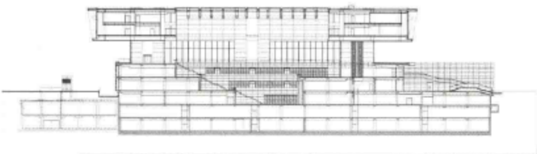
纵向截面图1
