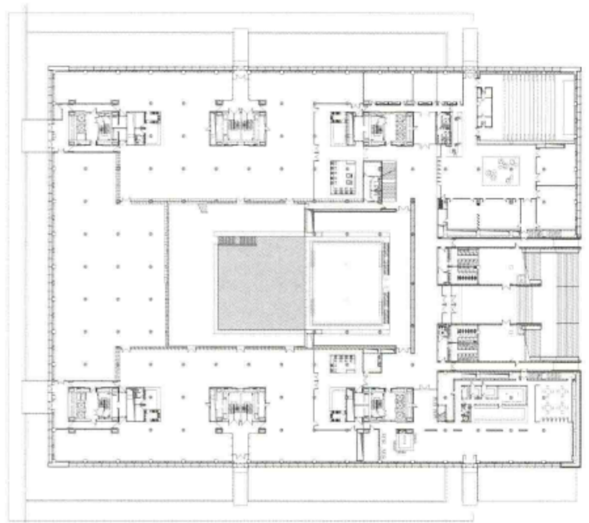
地面层平面图
