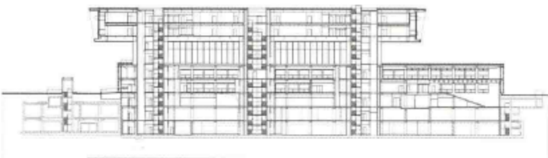
纵向截面图2
