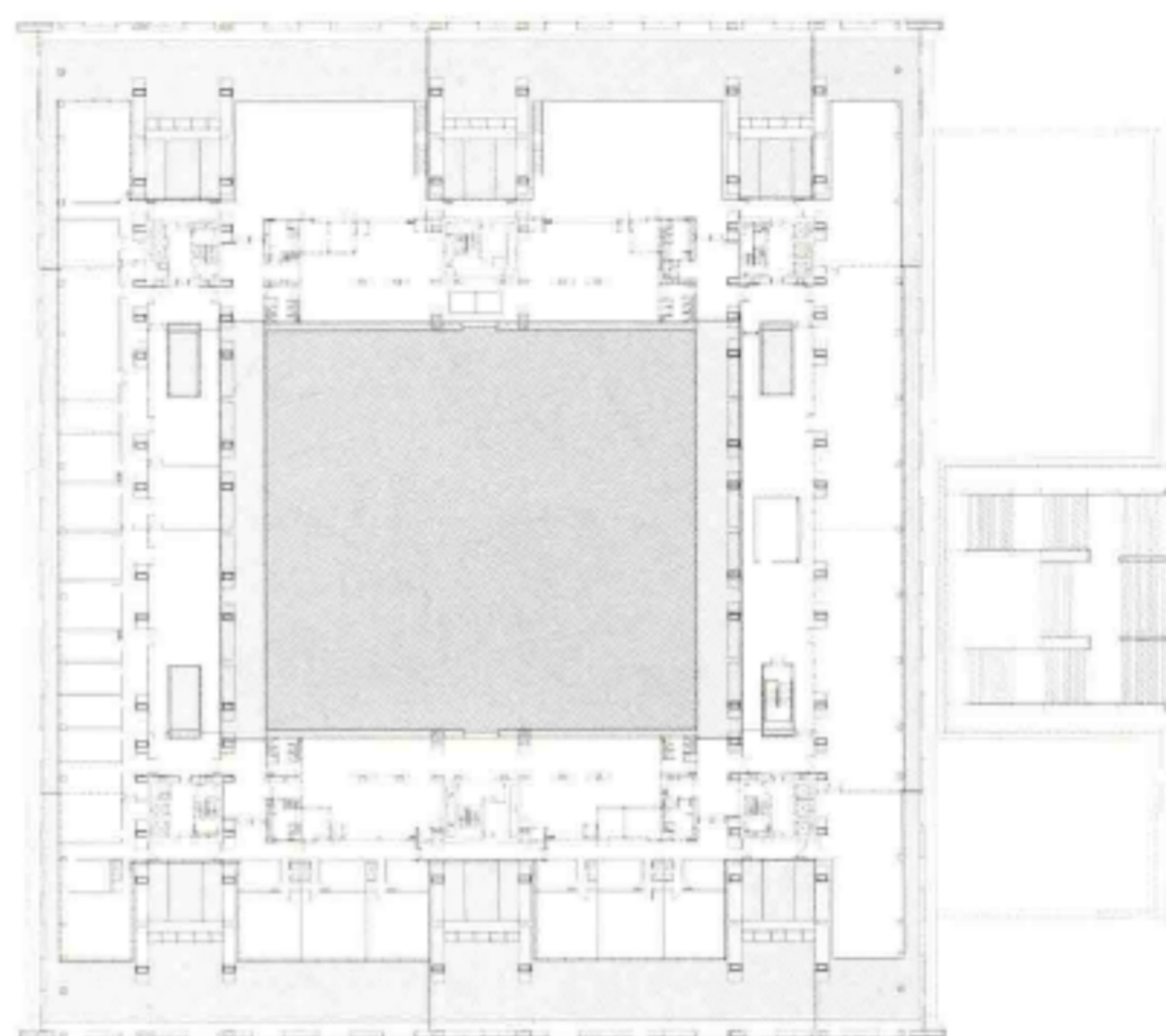
四层平面图
