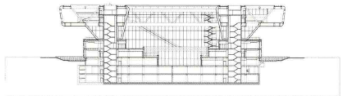
横向截面图1
