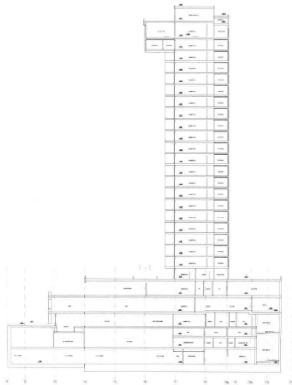
剖面图 B
