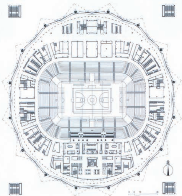
主体育馆二层平面
