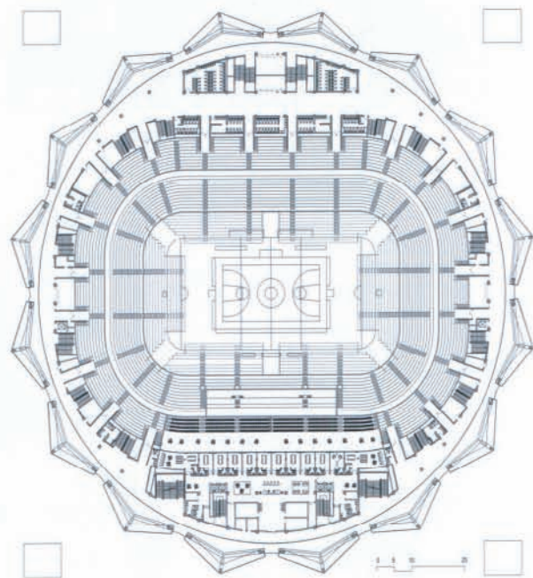
主体育馆三层平面
