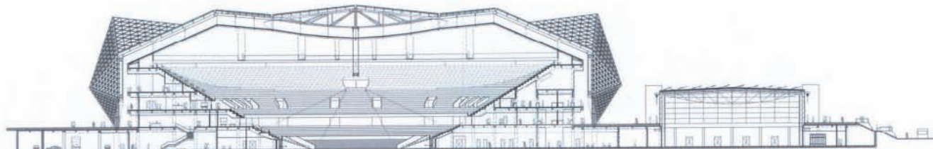
主体育馆剖面
