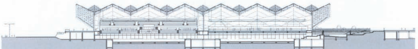
游泳馆剖面
